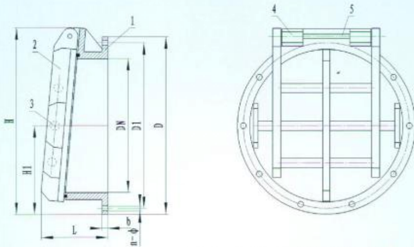
圆形衬钢HDPE拍门阀装配示意图
