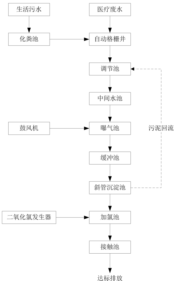
图 1 污水处理站工艺流程图
